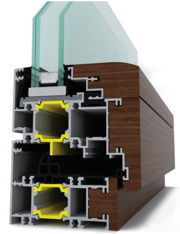
altimba 89 U_{min} : 1,31 \text{ W/m}^2\text{K}
