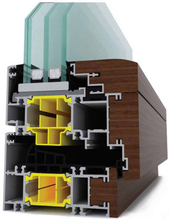
altimba 99 U_{min} : 0,90 \text{ W/m}^2\text{K}
